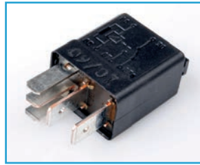
PRZEKAŹNIK MINIATU- ROWY 12V 5–styk. zwier.-rozw. 20/10A
