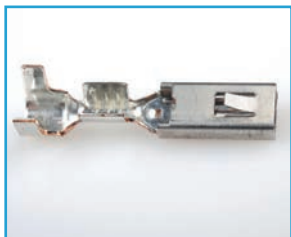
KOŃCÓWKA żeńska seria 2,8 DS zast. Opel, inne ➤ nr kat. 391 Opakowanie 1 kpl. (10szt.)
