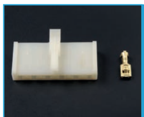
ZŁĄCZE TYLNEJ LAMPY (6x4,8/1,5) PN Caro 6-styk.
