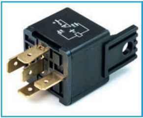
PRZEKAŹNIK 5–styk. sam. 561/4120 12V 30/40 AMP
