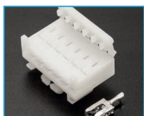
ZESTAW 6–styk. LAMPY DUCATO > nr kat. 1109 Opakowanie 1 kpl. (1x O+K)
