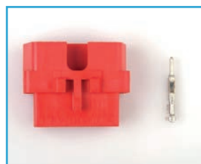
GNIAZDO DIAGNOSTYCZNE czerwone 16-styk.
