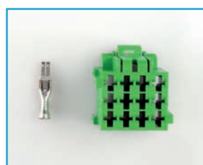
Obudowa żeńska SICMA 1,5 12-styk.
